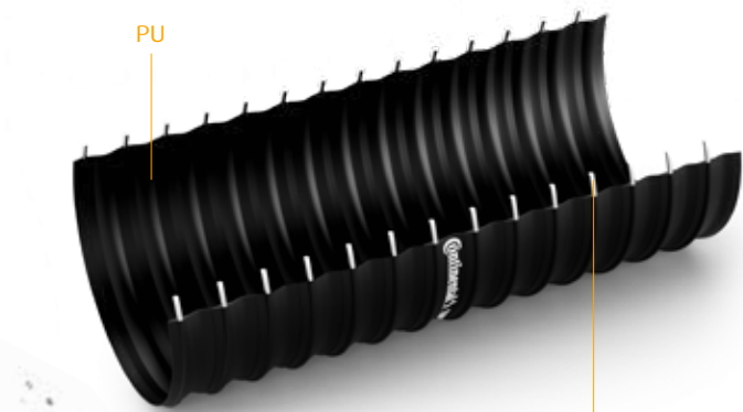
Konduktiv PU-belagd kopparbelagd stålspiral. Conductive PU coated galvanised steel spiral
