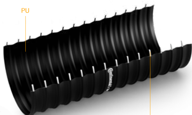
Leitfähige, PU-ummantelte, verzinkte Stahlspirale Conductive PU coated galvanised steel spiral
