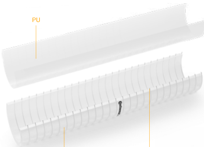
Terässpiraali Steel spiral
